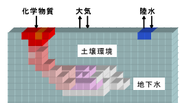
GERAS-3(3次元数値解析モデル) 浄化効果等を加味した詳細モデル
