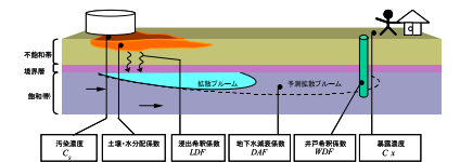
GERAS-2(2次元モデル) サイト固有の評価モデル
