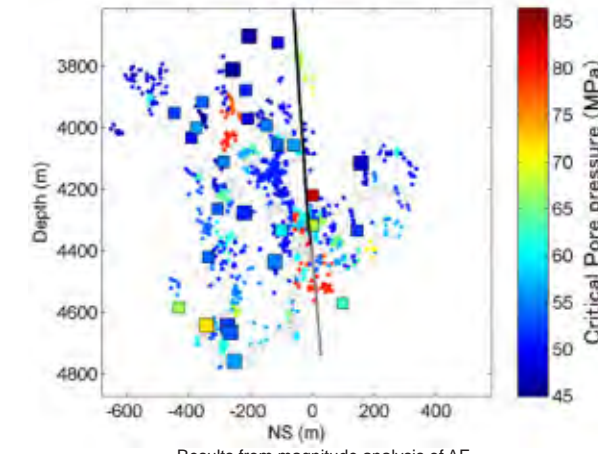
Results from magnitude analysis of AE 貯留層内臨界間隙水圧分布とAEマグニチュードの関連性(スイス、バーゼル)
