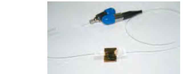
図4：MEMS技術により作製した、光干渉型ハイドロフォン（上）およびSPRセンサ（下）
