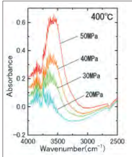
超臨界環境での薄膜水の赤外吸収スペクトル
