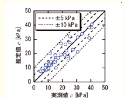
図3 粘着力 c の実測値(一面せん断試験結果)とBPNNによる推定値の比較結果
