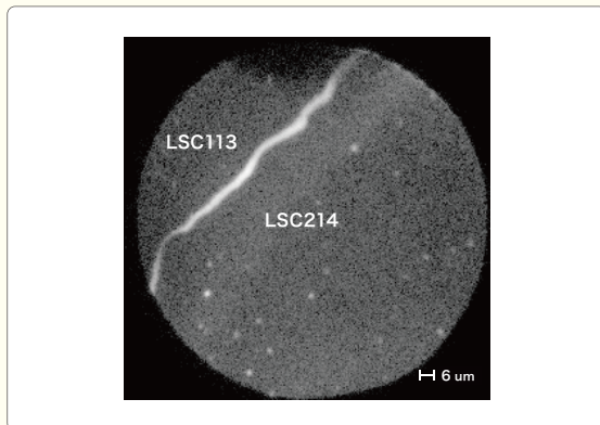
図1 酸素同位体 18 Oを利用したLSC214/LSC113ヘテロ界面における酸素取込反応の可視化
