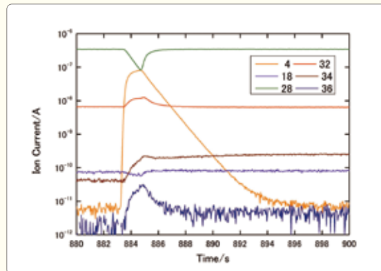
図2 パルス同位体交換法によるLSC113粉末試料の酸素取込反応評価 (500°C, 0.05%O 2 )
